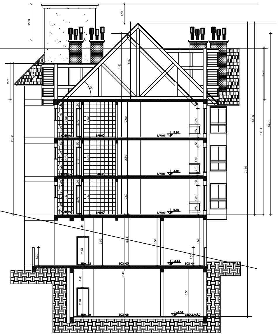
CORTE B B Esc.: 1/75
