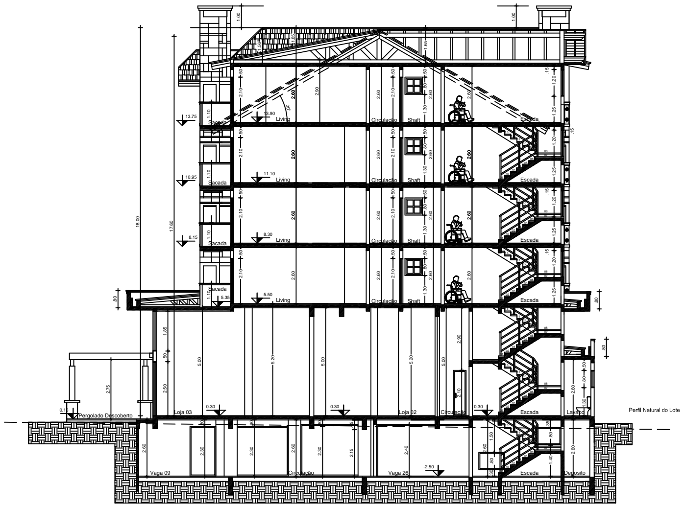
CORTE AA
