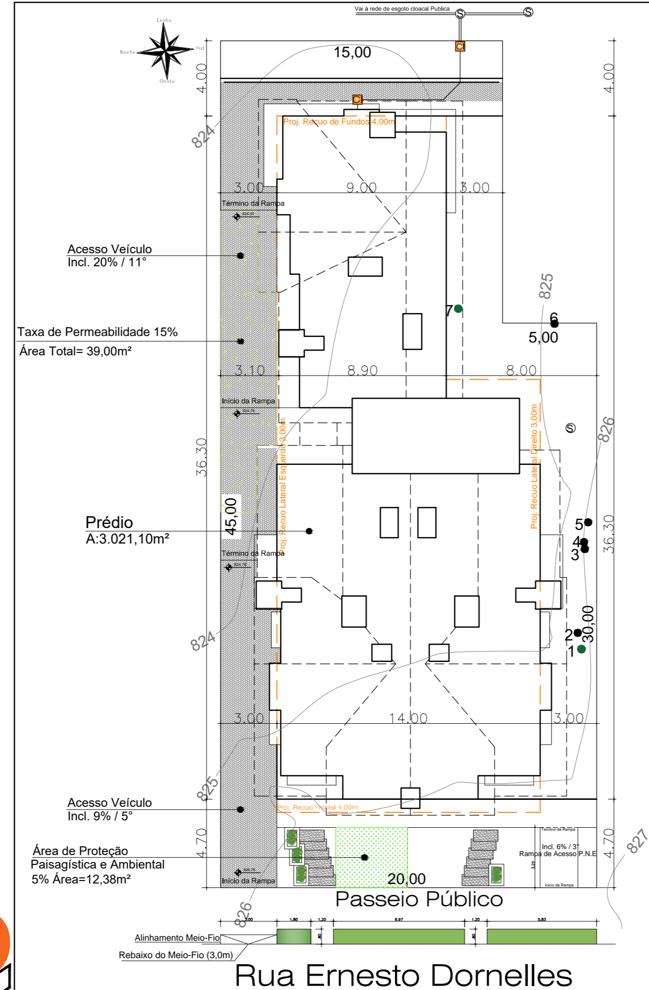
Planta de Situação Localização Esc: 1/200
